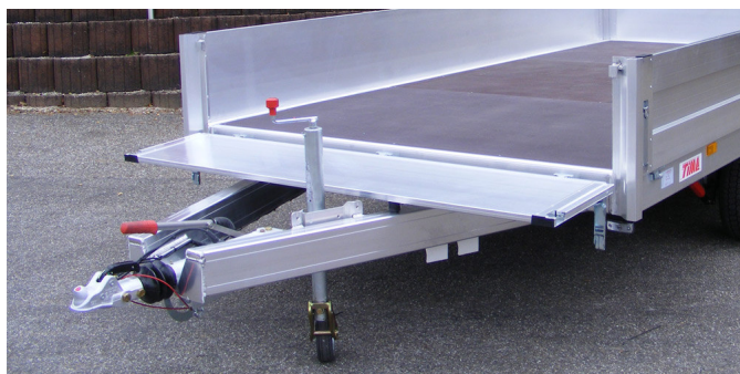
Stirnwand abgeklappt
