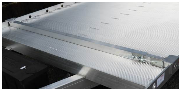
einteilige Auffahrrampen in Fahrstellung
